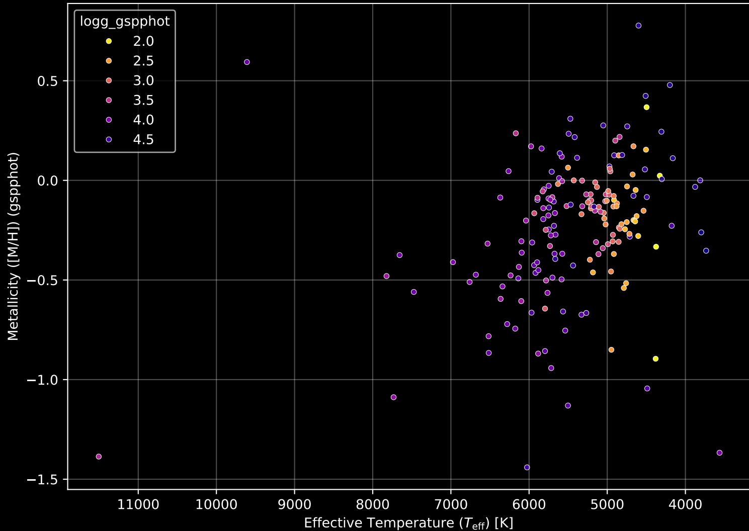
APOGEE DR17 Field: [266-26-O_TESS] Stellar Population Parameters (n= 179)
